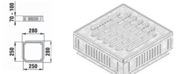
TERRAFIX POINT TYPE 25/25, hauteur réglable 70-100 mm, 250x250 mm Collecteur type 25/25 avec grille passerelle, fentes 136-186x10, galva
