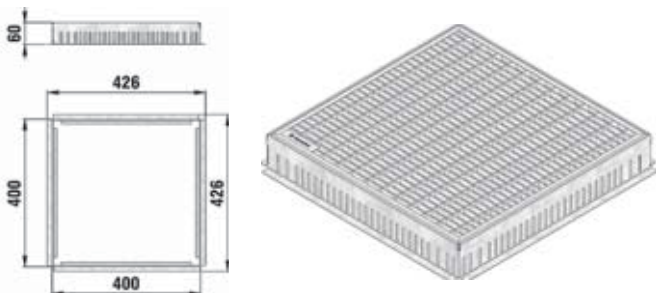
TERRAFIX POINT TYPE 40/40, hauteur fixe 60 mm, 400x400 mm Collecteur type 40/40 avec caillebotis, mailles 30x10, galva
