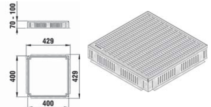
TERRAFIX POINT TYPE 40/40, hauteur réglable 70-100 mm, 400x400 mm Collecteur type 40/40 avec grille caillebotis, mailles 30x10, galva
