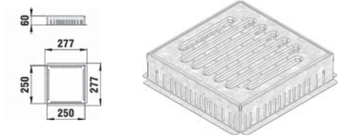
TERRAFIX POINT TYPE 25/25, hauteur fixe 60 mm, 250x250 mm Collecteur type 25/25 avec grille passerelle, fentes 136-186x10, galva
