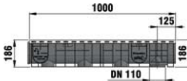
Type 010, vue détaillée
